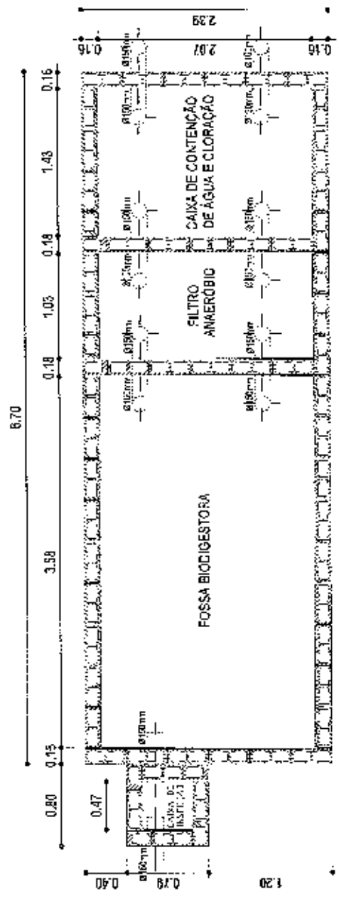
PLANTA BAIXA TOBOAGUA ESC 1/25
